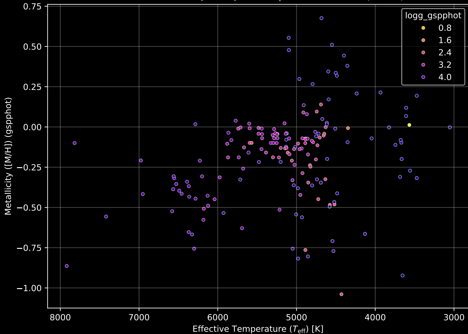
APOGEE DR17 Field: [150-45] Stellar Population Parameters (n= 174)
